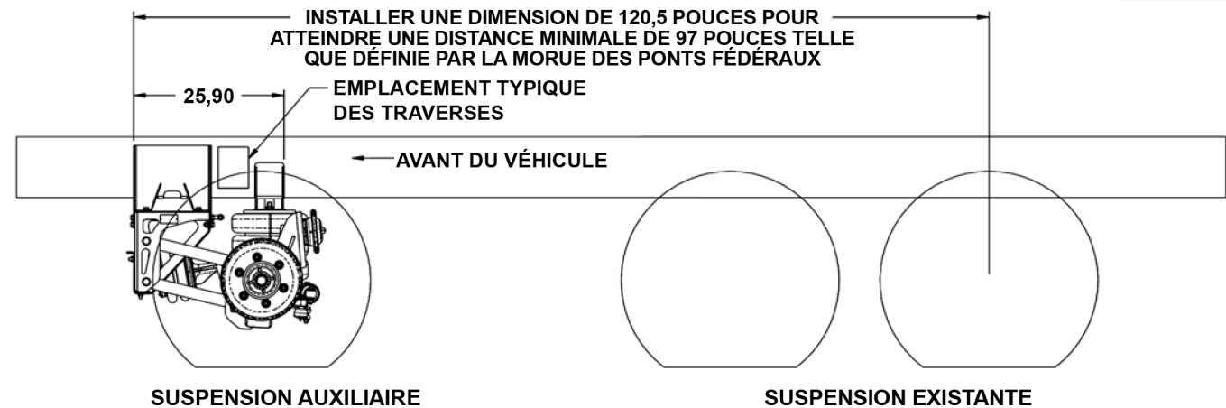
CONFIGURATION DU POUSSOIR
